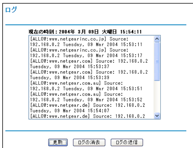
図 5-5: ログ画面
