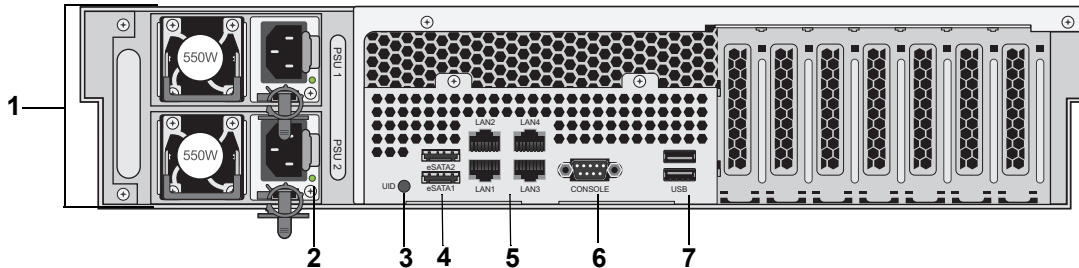
図 11. 3220 の背面
