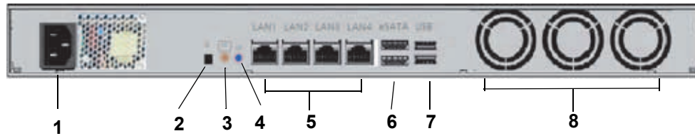
図 7. 背面
