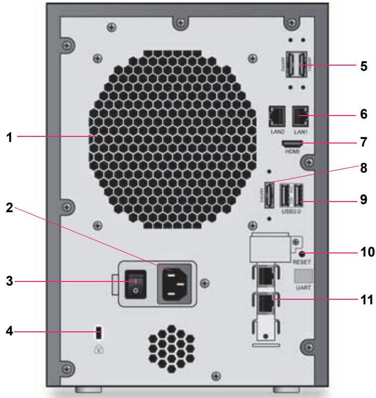
図 21. ReadyNAS 716X の背面
