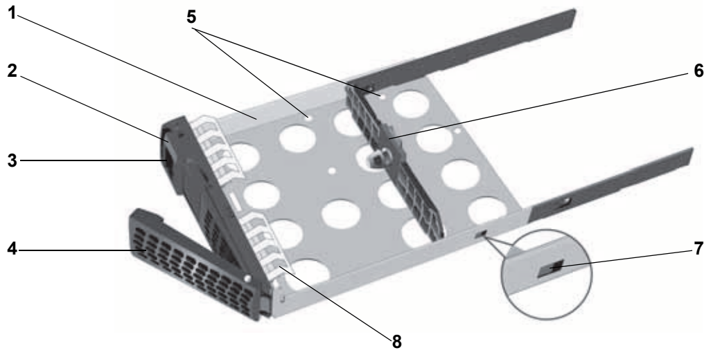
図 26. EDA 500 ディスクトレイ
