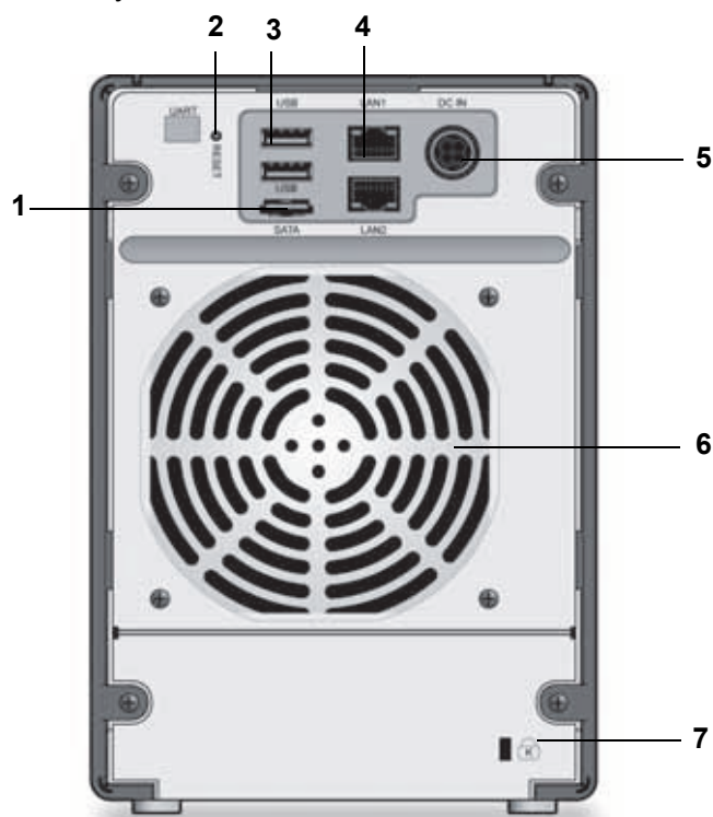
図 6. ReadyNAS 104 の背面
