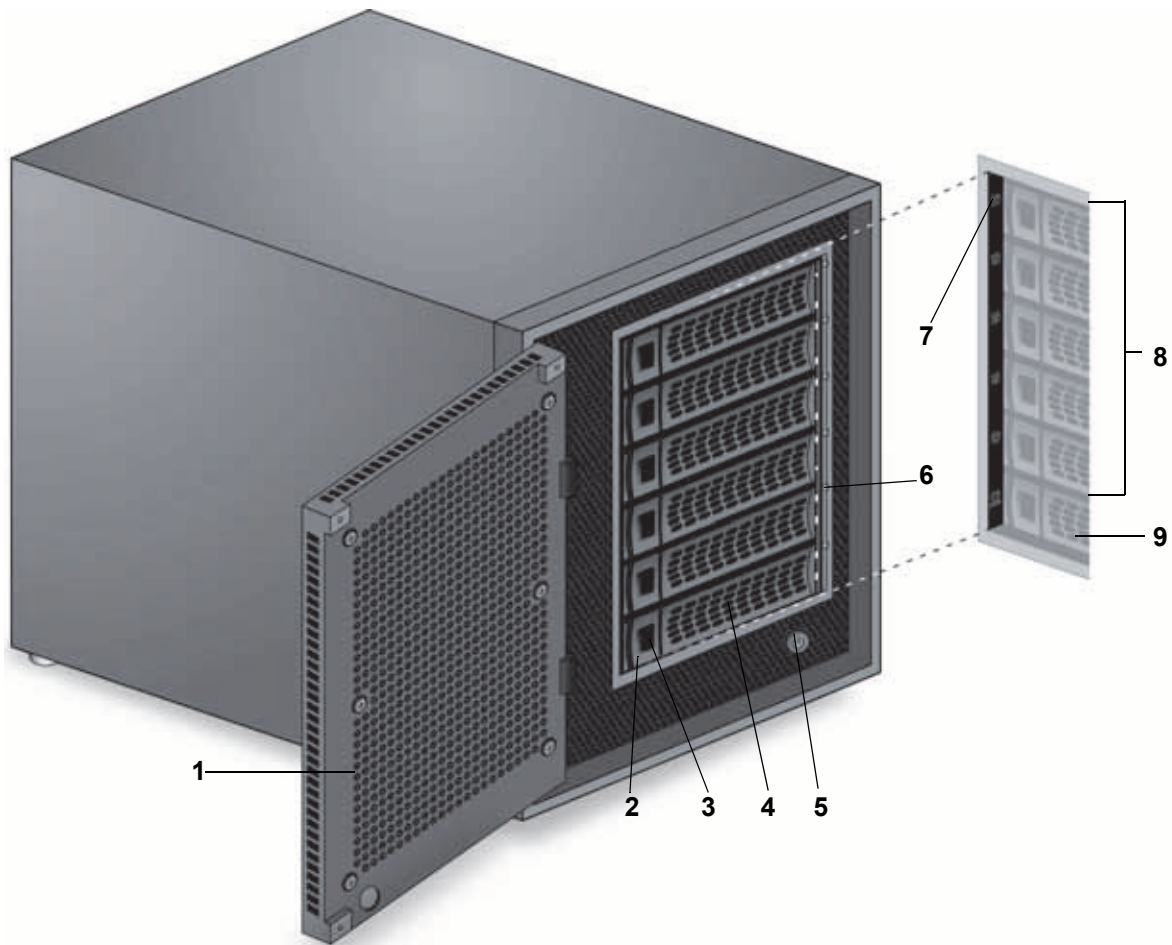
図 23. EDA 500 のドライブベイ
