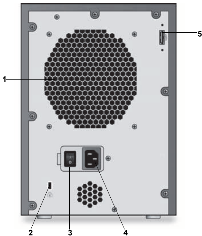
図 24. EDA 500 の背面
