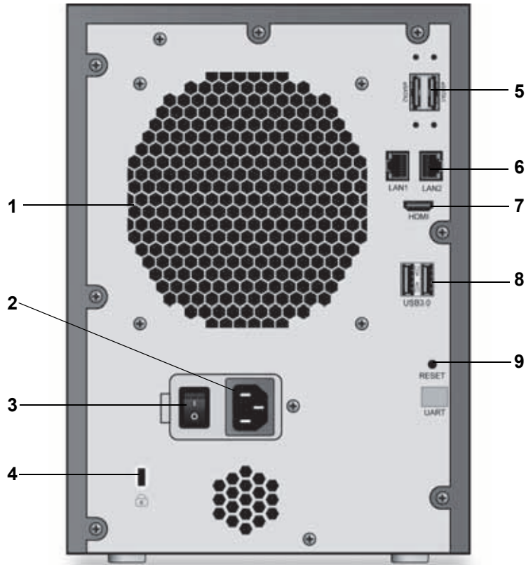
図 15. ReadyNAS 316 の背面
