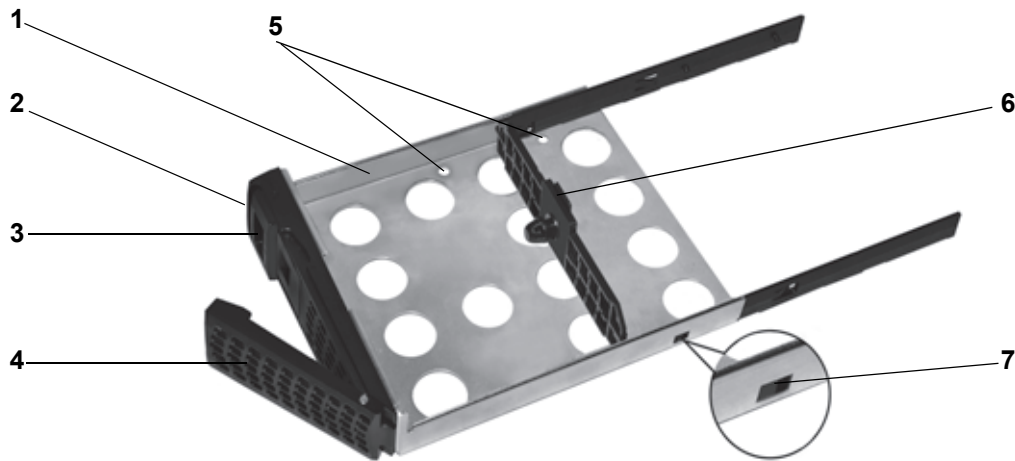
図 25. 標準ディスクトレイ
