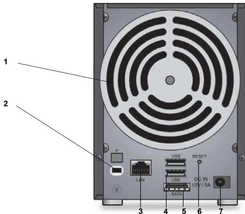
図 3. ReadyNAS 102 の背面
