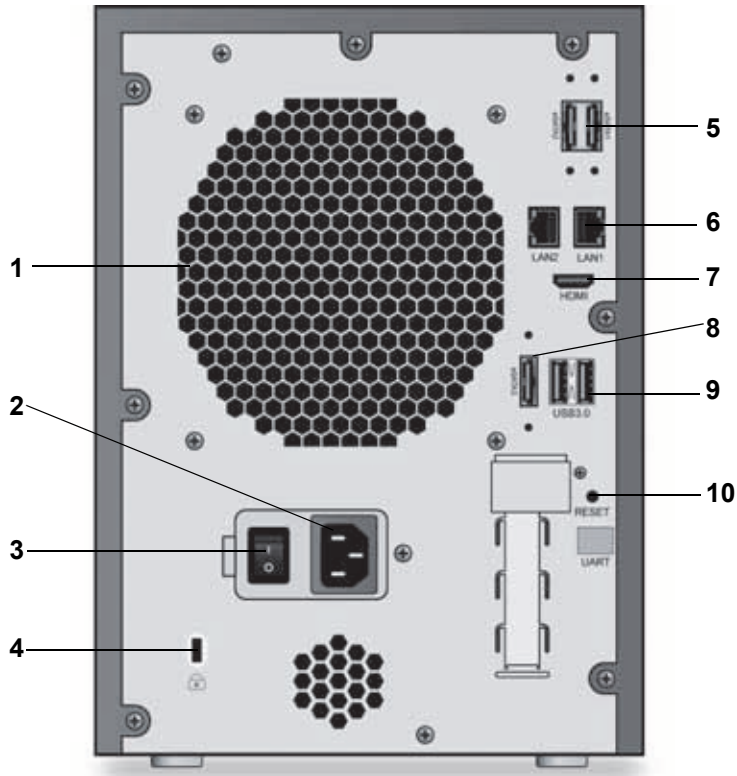
図 18. ReadyNAS 516 の背面
