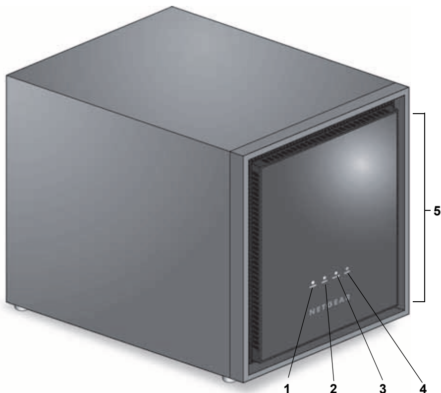
図 22. EDA 500 の前面と側面
