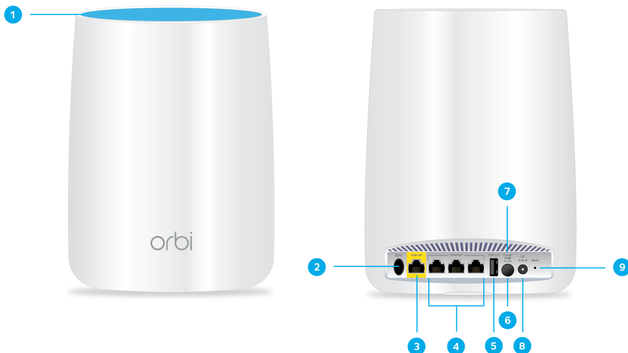
図 2 : OrbiルーターモデルRBR50の前面および背面
