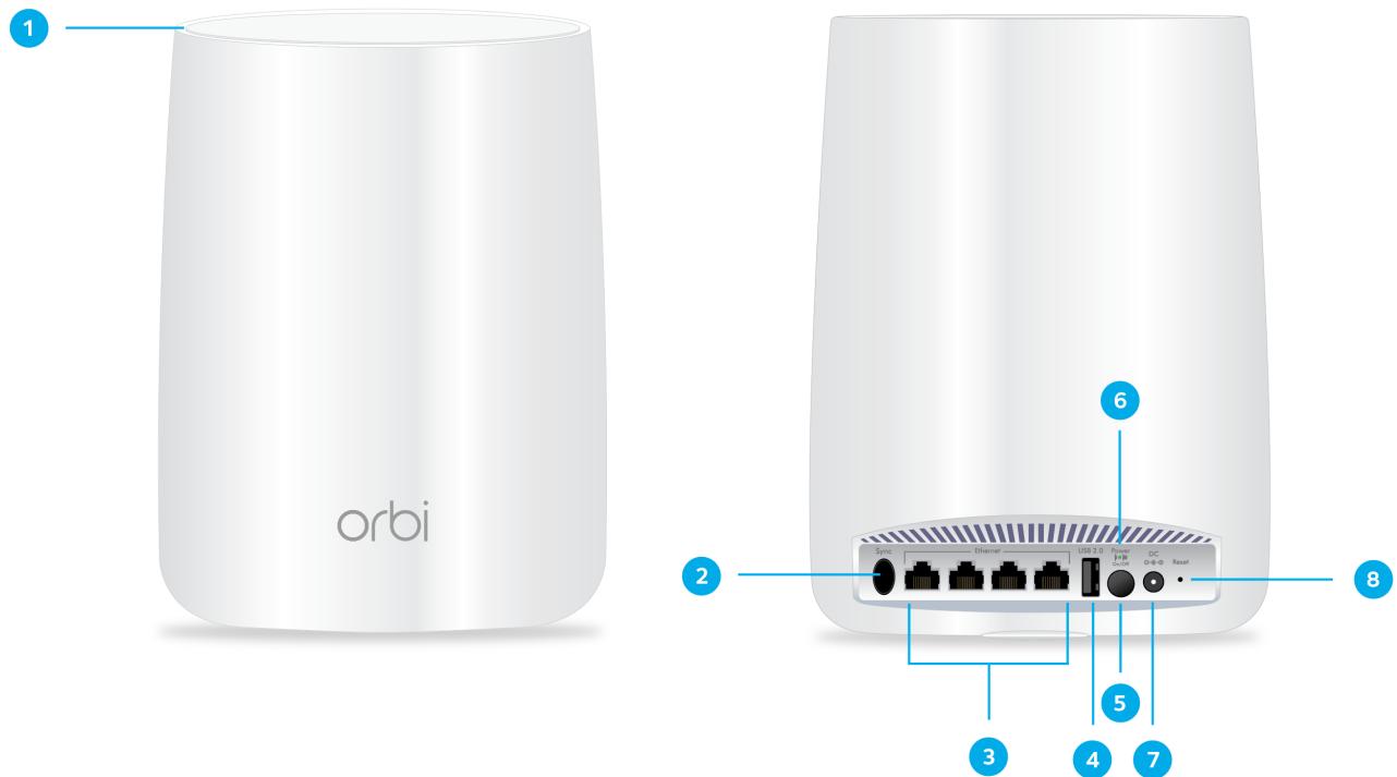
図 3 : OrbiサテライトモデルRBS50の前面および背面
